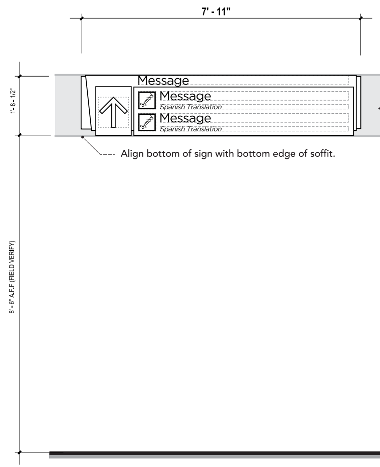
6 ELEVATION - SOFFIT SCALE: 1/2" = 1' - 0"
