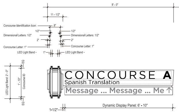
1 TOP VIEW - SOFFIT SCALE: 1/2" = 1' - 0"
