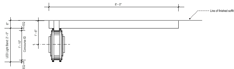
1 TOP VIEW - SOFFIT SCALE: 1/2" = 1' - 0"
