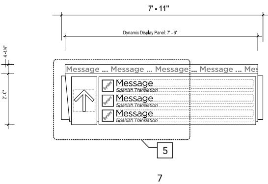
1 TOP VIEW SCALE: 1/2" = 1' - 0"
