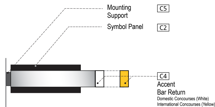
6 TOP VIEW SCALE: 1-1/2" = 1' - 0"
