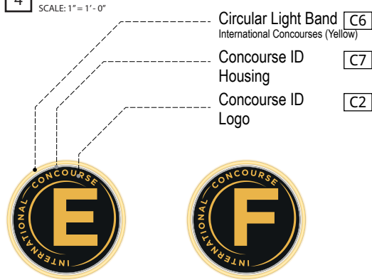
4 SIGN FINISHES SCALE: 1" = 1' - 0"
