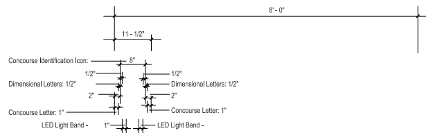
1 TOP VIEW - SOFFIT SCALE: 1/2" = 1' - 0"
