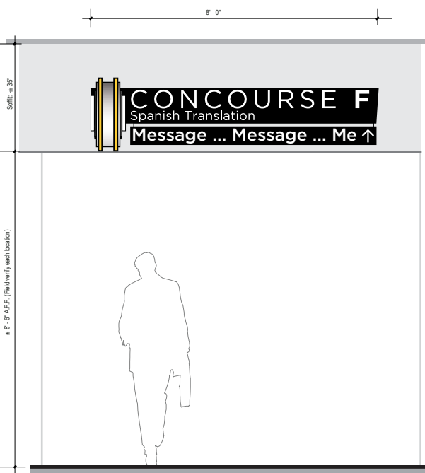
8 ELEVATION SCALE: 1/2" = 1' - 0"
