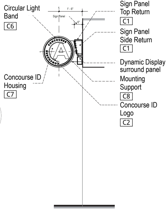
6 END VIEW - 1 SCALE: 1/2" = 1' - 0"
