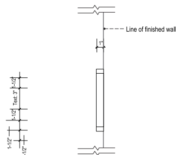
3 SIDE VIEW SCALE: 1-1/2" = 1' - 0"
