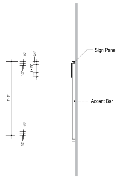
3 SIDE VIEW SCALE: 1 - 1/2" = 1' - 0"
