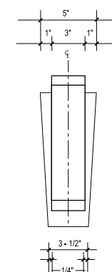
3 SIDE VIEW SCALE: 1-1/2" = 1' - 0"
