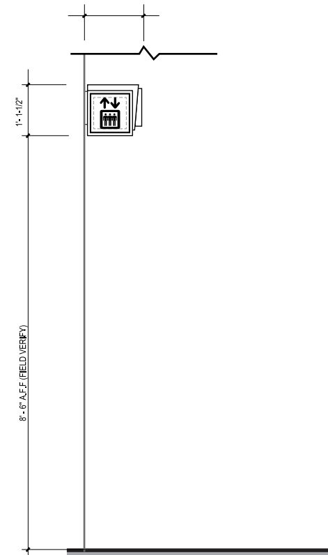
7 ELEVATION SCALE: 1-1/2" = 1' - 0"
