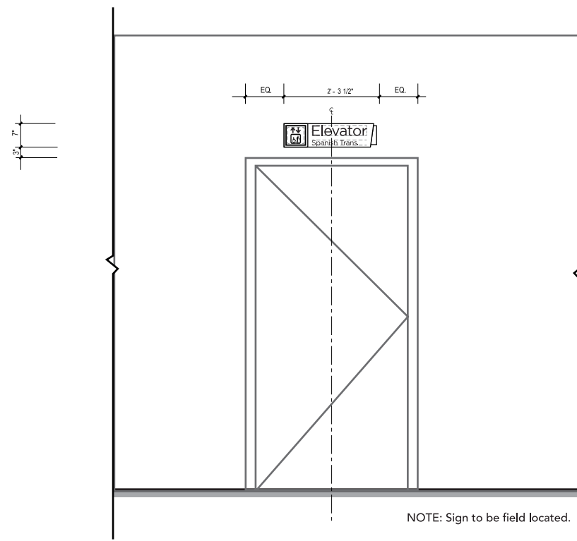
9 ELEVATION SCALE: 1/2" = 1' - 0"
