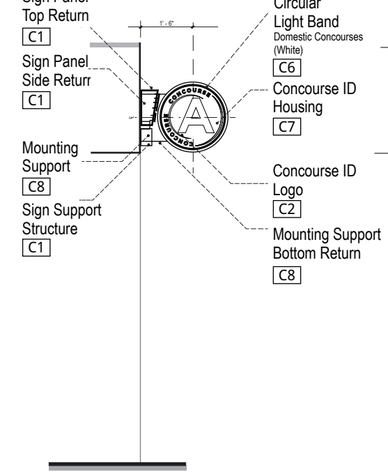
7 END VIEW - 2 SCALE: 1/2" = 1' - 0"
