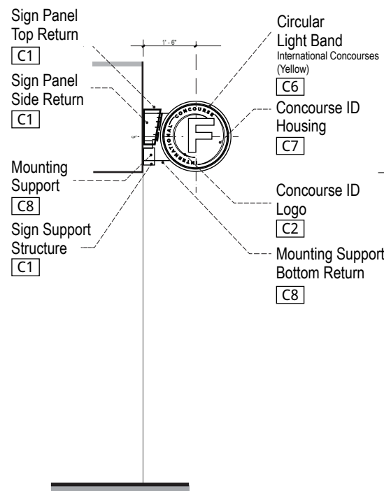
7 END VIEW - 2 SCALE: 1/2" = 1' - 0"
